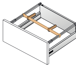
ПОПЕРЕЧНИЙ РЕЙЛІНГ ДЛЯ ATIRA / CROSS RAIL FOR TANDEMBOX/ATIRA
