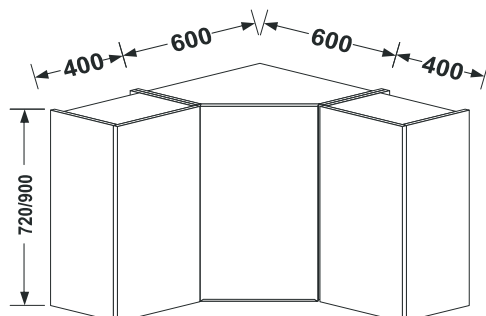
БЕРХНІ СЕКЦІЇ / UPPER SECTIONS
