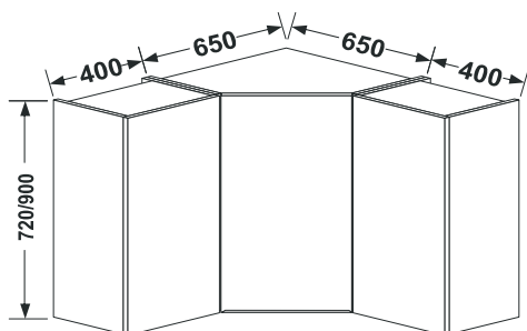
БЕРХНІ СЕКЦІЇ / UPPER SECTIONS
