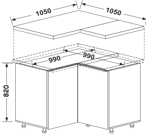
НИЖНІ СЕКЦІЇ / LOWER SECTIONS
