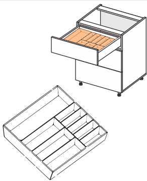
ЛОТОК ДЛЯ СТОЛОВИХ ПРИБОРІВ / CUTLERY TRAY
