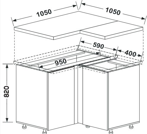
НИЖНІ СЕКЦІЇ / LOWER SECTIONS
