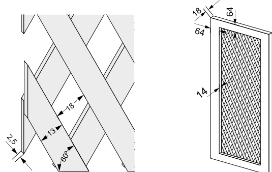
Схема ДЕКОРАТИВНОЇ РЕШІТКИ
