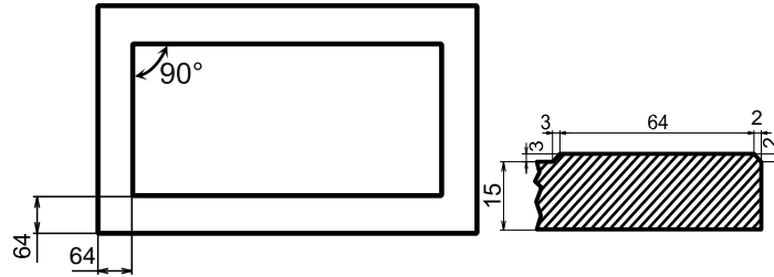
Схема фасада ДОМІНІ
