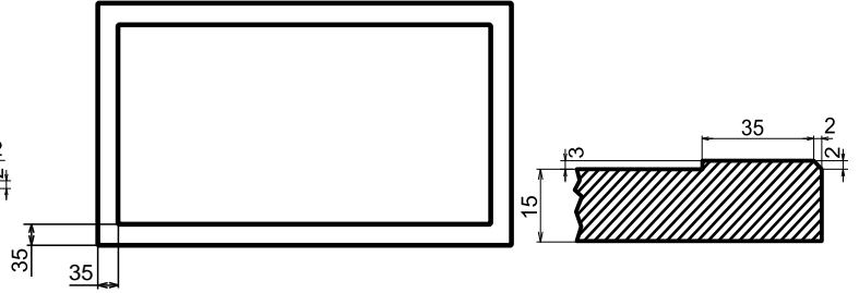
Схема рамочного профілю ВІТАЖ +
