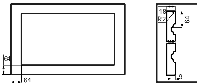
Схема фасада ВІЛСОН
