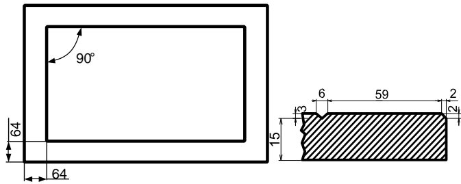
Схема рамочного профілю ВІТАЖ +
