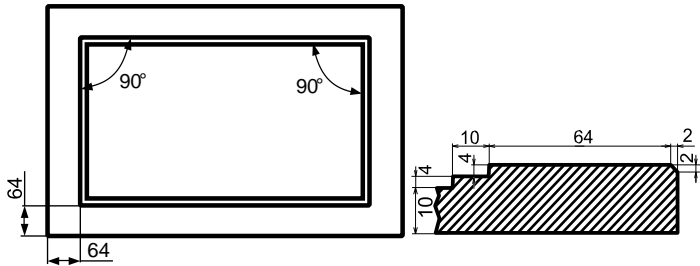
Схема фасада ВІЛСОН
